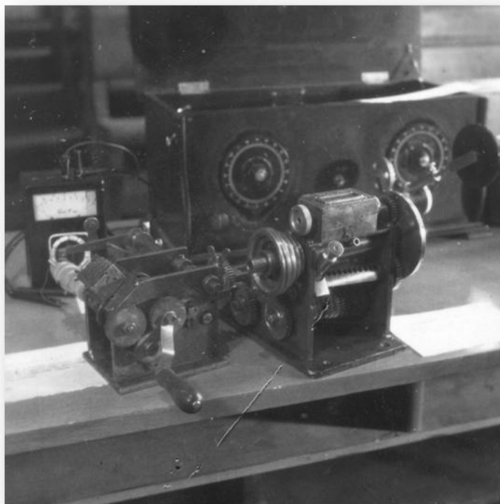
Obr. 8 Pozoruhodný exponát: amatérska navijačka krížovo vinutých cievok
